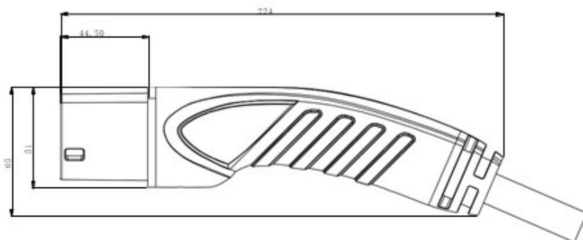
欧标枪端插头外形图
